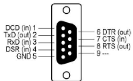
DB9 (гнездо)
