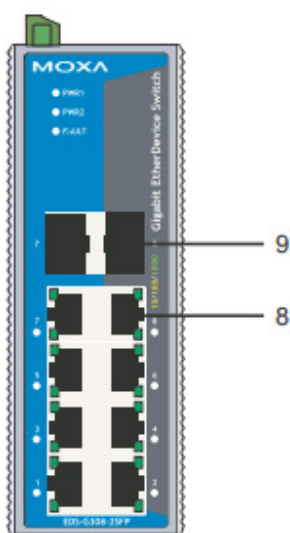
Передняя панель
