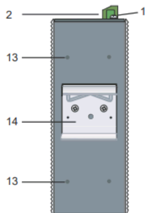
Вид сзади
