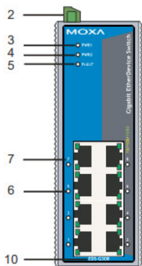
Передняя панель
